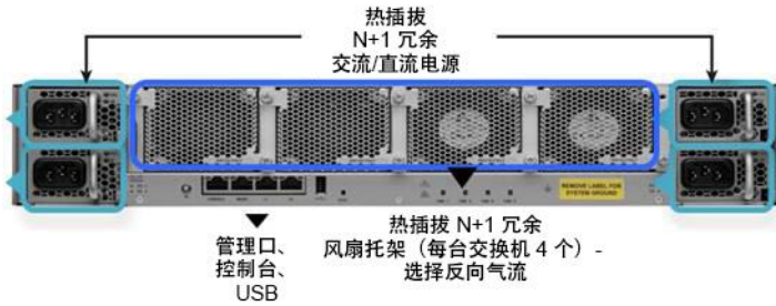
图 7. Cisco Nexus 56128P 交换机（风扇侧视图）
