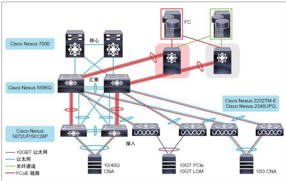
图 12. 多跳 FCoE 设计
