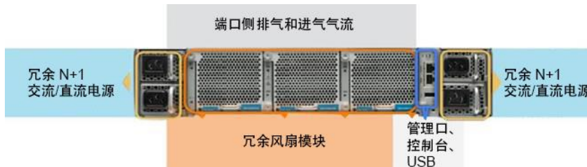
图 5. Cisco Nexus 5648Q 交换机（风扇侧视图）
