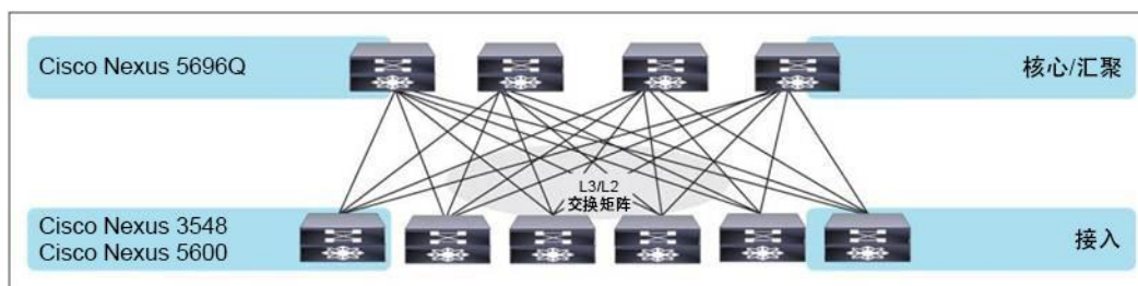
图 13. 高性能计算设计
