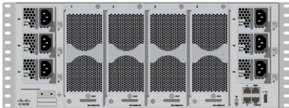
图 10. Cisco Nexus 5696Q 交换机（风扇侧视图）
