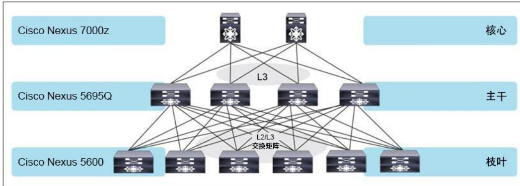
图 11. 枝叶和主干架构
