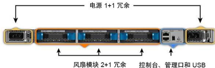
图 3. Cisco Nexus 5624Q 交换机（风扇侧视图）
