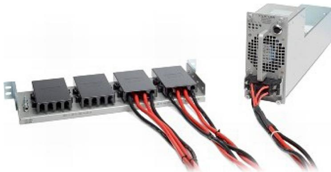
图 4. Cisco Nexus 7000 系列直流 PIU
