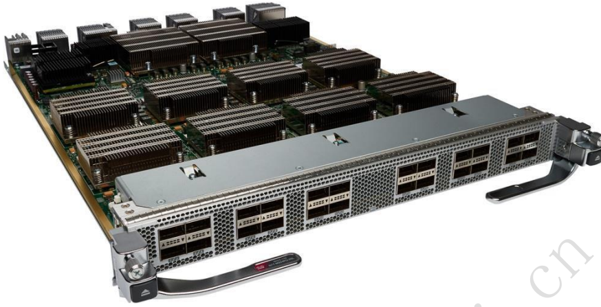
图 1. Cisco Nexus 7700 M3 系列 24 端口 40 千兆以太网模块
